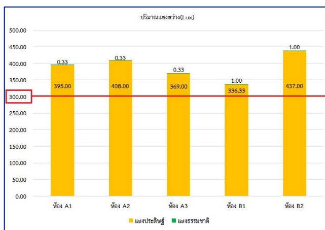
รูปภาพที่ 8 แสดงค่าเฉลี่ยความสว่าง (Illuminance) ห้องเรียนขนาดใหญ่
