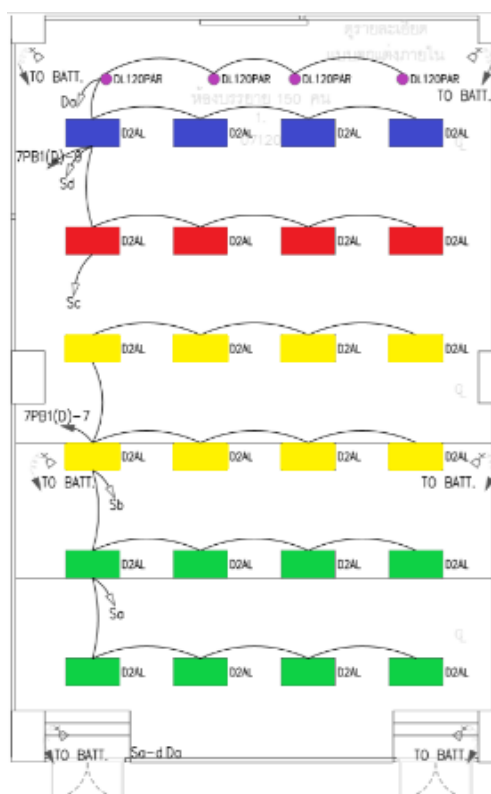
รูปภาพที่ 10 แสดงรูปแบบการแบ่งสวิตช์เปิด-ปิดดวงโคม
