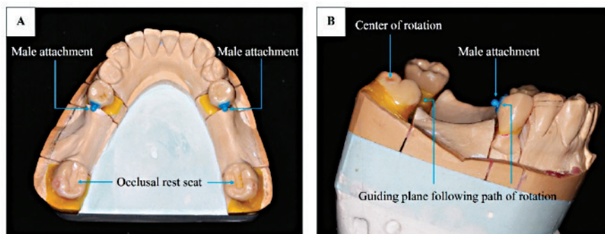
รูปที่ 20 การติดสลักยึดตัวผู้ที่ด้านใกล้กลางของฟันหลักด้านหน้าสันเหงือกกว้างบนระนาบนำตามวิธีการหมุน A: มุมมองด้านบนเคี้ยว B: มุมมองด้านข้าง
