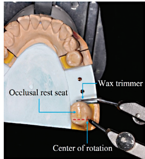
รูปที่ 14 มุมมองด้านบดเคี้ยวของแบบจำลองฟันหลัก ที่ตำแหน่งท้ายสุดของแอ่งรับส่วนพักด้านบดเคี้ยว (เส้นประสีแดง) ต้องตรงกับตำแหน่งจุดศูนย์กลางการหมุน (จุดสีแดงด้านแก้มใกล้กลางของฟันหลัก)
