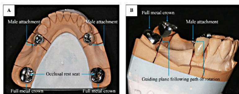
รูปที่ 21 ครอบฟันหลักซี่ 35 45 (ฟันหลักด้านหน้า) 38 และ 48 (ฟันหลักด้านหลัง) ภายหลังจากหล่อโลหะ โดยที่ครอบฟันซี่ 35 และ 45 มีสลักยึดตัวผู้ติดอยู่ที่ระนาบนำตามวิธีการหมุน A: มุมมองด้านบนเคี้ยว B: มุมมองด้านข้าง
