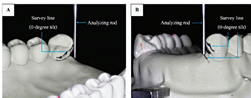
รูปที่ 29 การสำรวจแบบจำลองฟันหลักที่ตำแหน่งระนาบบดเคี้ยวขนานกับแนวระนาบจะปรากฏส่วนคอดที่ต้องปิดในปริมาณมากหากออกแบบฟันเทียมบางส่วนถอดได้แบบปกติที่มีแนวการถอดใส่ที่ตั้งฉากกับระนาบบดเคี้ยว
