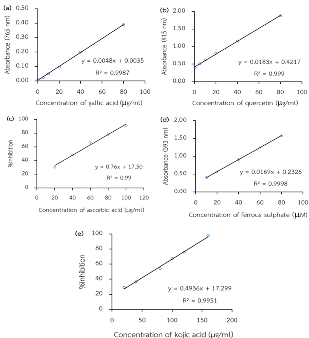
ภาพ 1 ตัวอย่างกราฟมาตรฐาน (a) gallic acid จากการทดสอบ TPC (b) quercetin จากการทดสอบ TFC (c) ascorbic acid จากการทดสอบ DPPH (d) ferrous sulphate จากการทดสอบ FRAP และ (e) kojic acid จากการทดสอบ dopachrome
