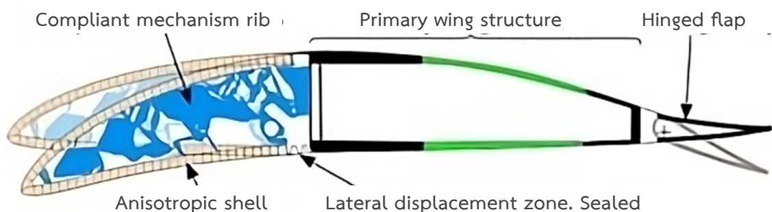
ภาพ 5 โครงสร้างของ Morphing Wing
