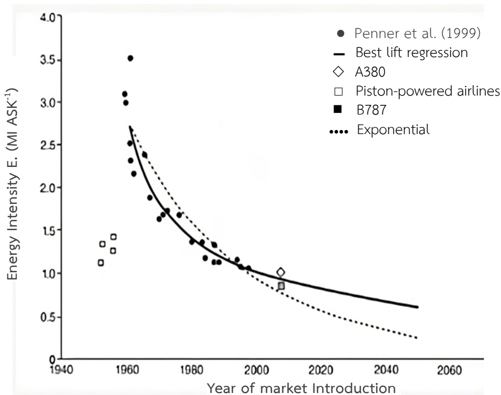
ภาพ 3 แนวโน้มความหนาแน่นของการใช้พลังงานในอุตสาหกรรมการบินตั้งแต่การเริ่มต้นของอุตสาหกรรมการบินพาณิชย์จนถึงการคาดการณ์ในปี ค.ศ. 2050
