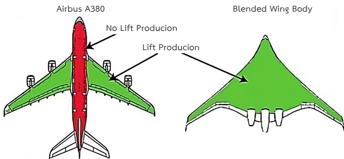
ภาพ 4 การเปรียบเทียบการสร้างแรงยกของเครื่องบินแบบ Airbus 380 และ Blended Wing-Body
