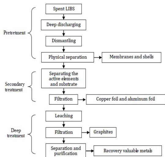
ภาพ 6 ขั้นตอนหลักสำหรับการ Recycle แบตเตอรี่ที่ใช้แล้วสำหรับยานยนต์ไฟฟ้า
