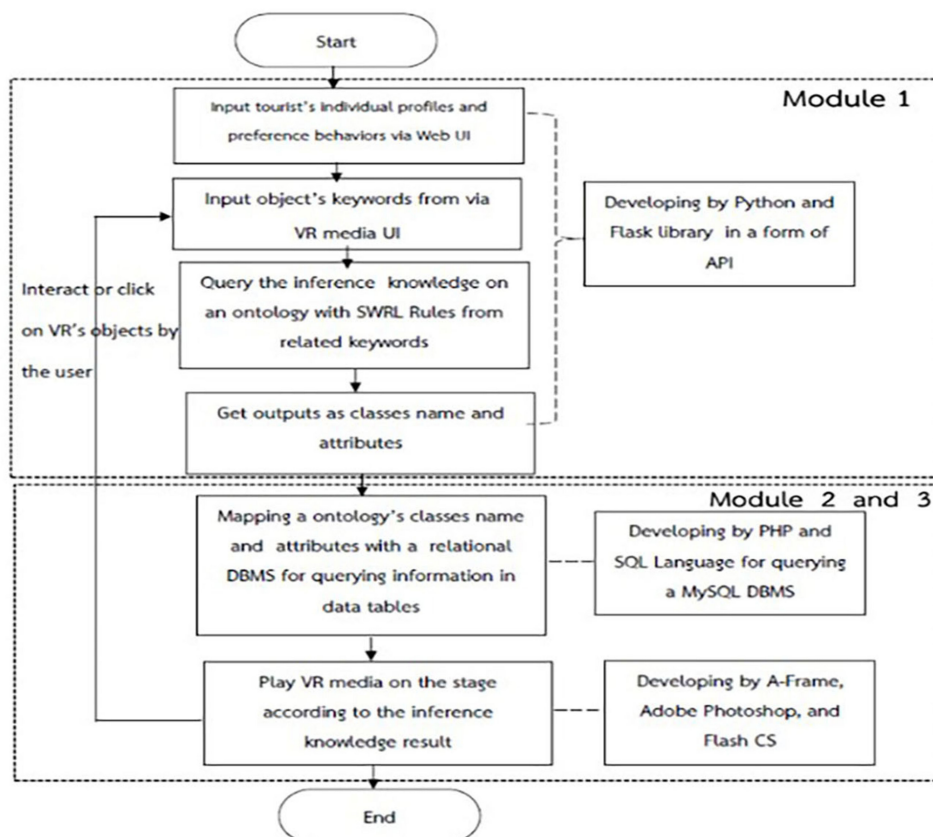
ภาพ 1 Flow chart ขั้นตอนวิธีการประมวลผลของสื่อความเป็นจริงเสมือนเชิงความหมาย
