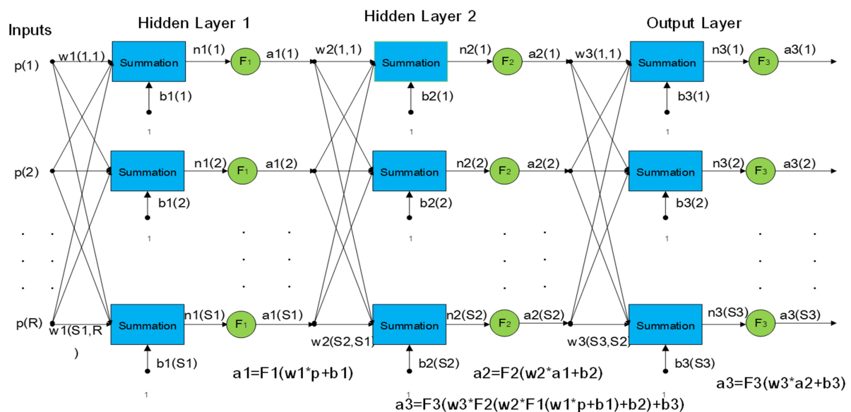
ภาพ 1 รูปแบบโครงข่ายประสาทเทียมสำหรับประยุกต์ใช้ในระบบไฟฟ้ากำลัง
