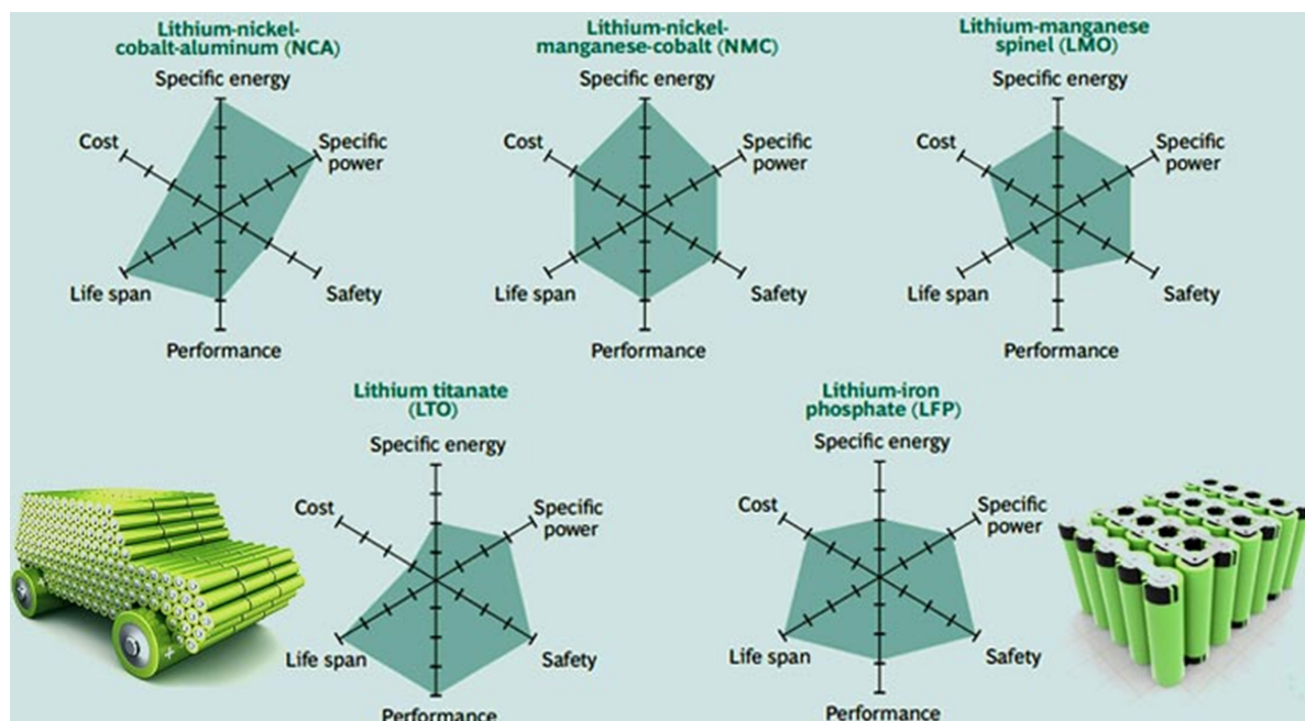
ภาพ 5 การเปรียบเทียบคุณสมบัติของแบตเตอรี่ลิเทียมไอออนแบบต่าง ๆ
