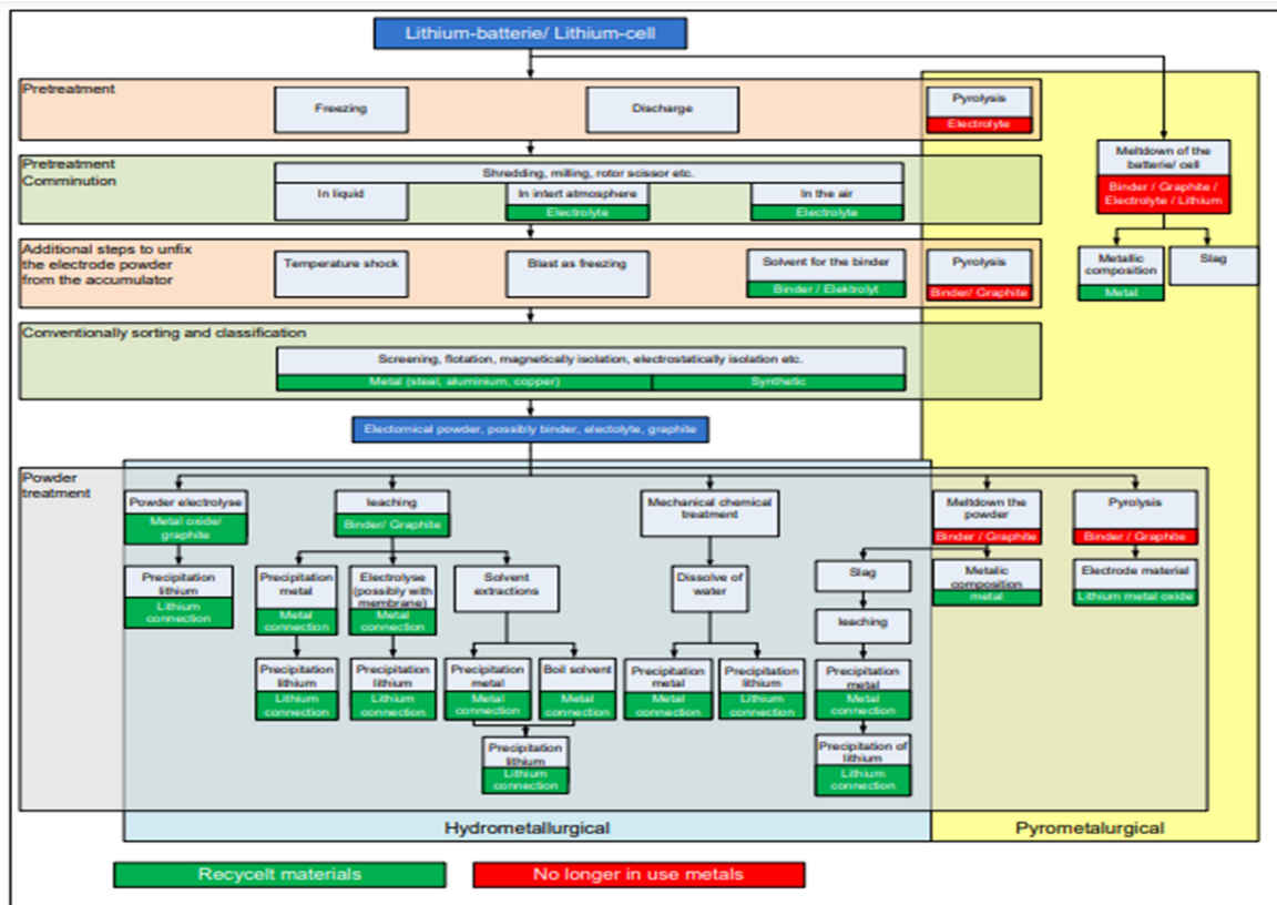
ภาพ 7 แสดงภาพรวมกระบวนการ Recycle แบตเตอรี่ลิเทียมไอออนสำหรับยานยนต์ไฟฟ้า
