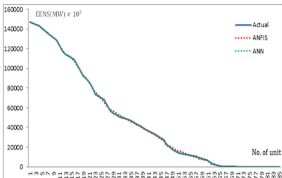
ภาพ 18 แสดงการเปรียบเทียบค่าพลังงานที่ไม่สามารถจ่ายของ โครงข่ายประสาทดเทียม ระบบอนุมานฟัซซีโครงข่ายปรับตัว ได้และค่าจริงสำหรับข้อมูลระบบผลิตด้วยความร้อน ของประเทศไทย Note. From Evaluation of Generation System Reliability Using Adaptive Neuro-Fuzzy Inference System (ANFIS) and Artificial Neural Networks (ANNs) by K. Wannakam and S.Jiriwibhakorn, 2018, International Review of Electrical Engineering (I.R.E.E.), 13(3), pp. 204-212 Copyright Praise Worthy Prize
