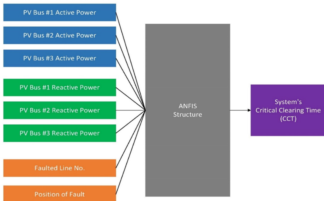
ภาพ 14 แสดงโครงสร้างอินพุตและเอาต์พุตสำหรับระบบอนุมานฟัซซี่โครงข่ายปรับตัว
