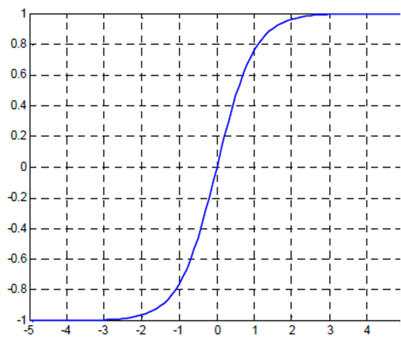
ภาพ 4 ฟังก์ชันถ่ายโอนแบบแทนจิมมอยด์
