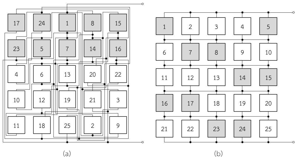
ภาพ 11 การบังเงาบางส่วน SW. a) การจัดเรียงโมดูลแบบเมจิกสแควร์ MS1; b) การกระจายเงาบางส่วน
