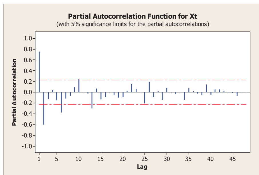
ภาพที่ 3 กราฟฟังก์ชันอัตโนมัติสหสัมพันธ์บางส่วน
